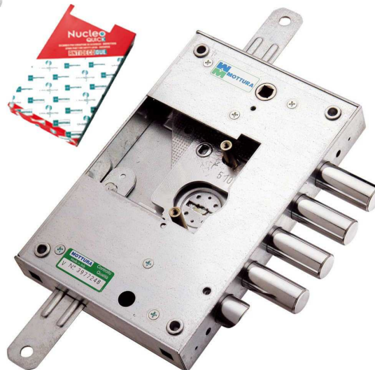
89NR471GRD CERRADURA MOTTURA GORJA CON NUCLEO 3 LLAVES DHA
